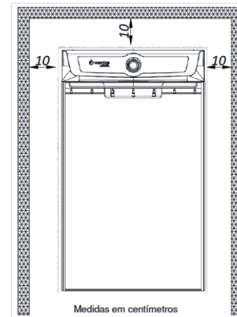
Distâncias Mínimas de Instalação
